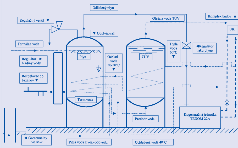
Schéma zapojenia kogeneračnej jednotky do systému s odplyňovačom
